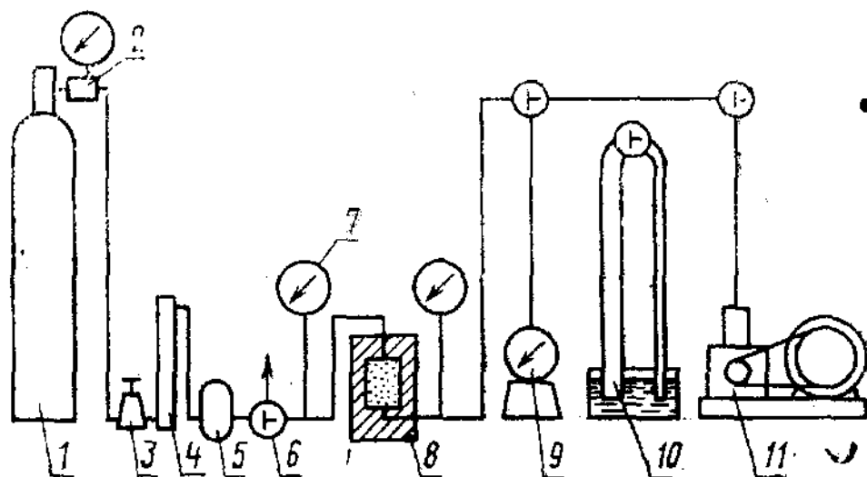
Принципиальная схема установки для определения газопроницаемости
